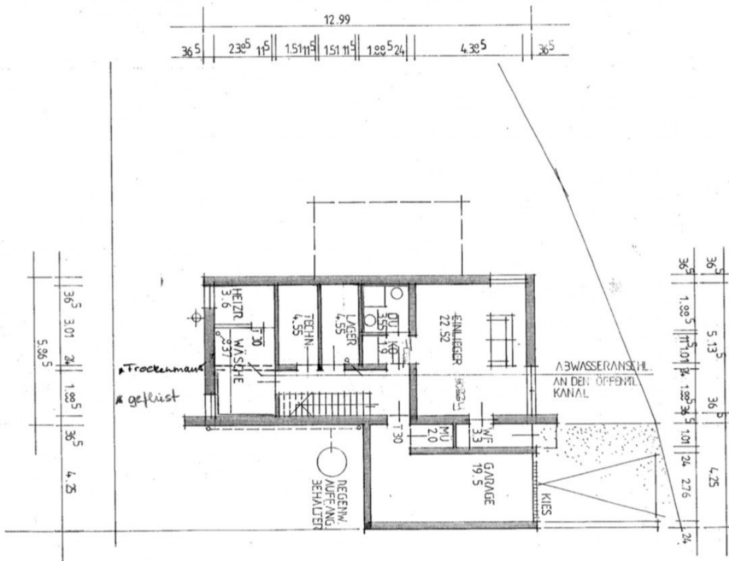
Grundriss Einliegerwohnung
